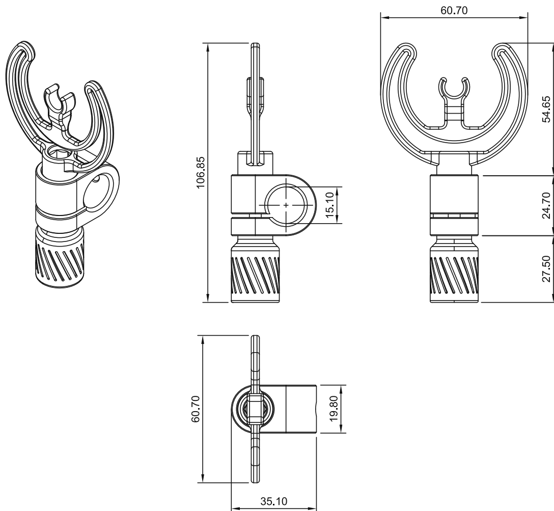
(EN) Lyre clamp kit dimensions (all dimensions in millimeters with \pm 0.2\text{mm} tolerance) (HR) Dimenzije kompleta stezaljke lire (sve dimenzije u milimetrima sa \pm 0.2\text{mm} tolerancijom)
