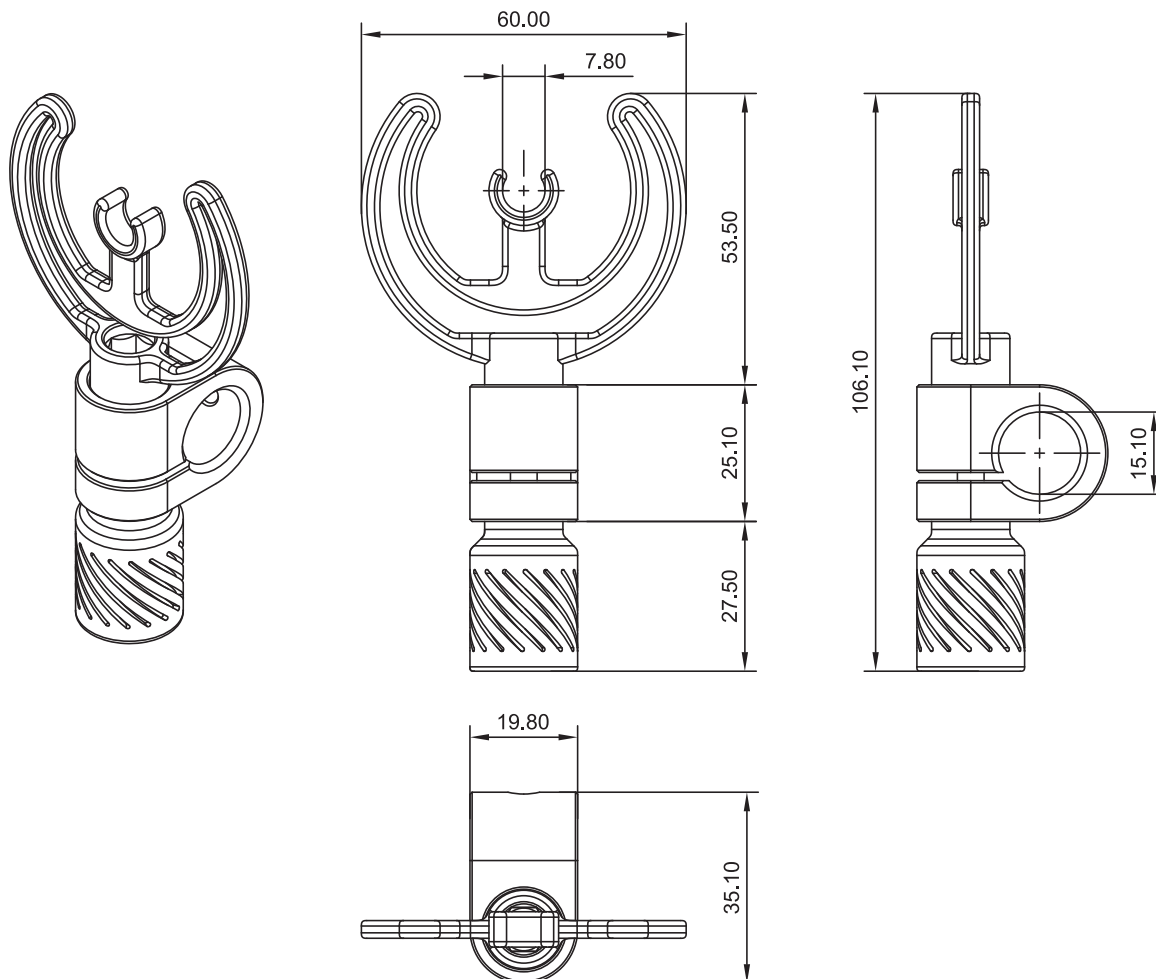
(EN) Lyre clamp kit dimensions (all dimensions in millimeters with \pm 0.2\text{mm} tolerance) (HR) Dimenzije kompleta stezaljke lire (sve dimenzije u milimetrima sa \pm 0.2\text{mm} tolerancijom)
